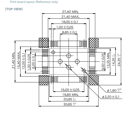
● プリント板レイアウト (参考図)
