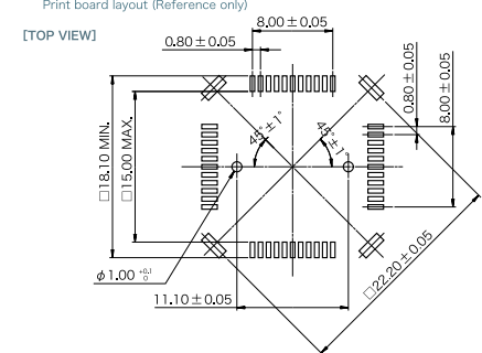
● プリント板レイアウト (参考図)
