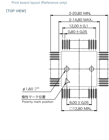
● プリント板レイアウト (参考図)
