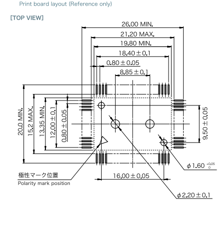
● プリント板レイアウト (参考図)
