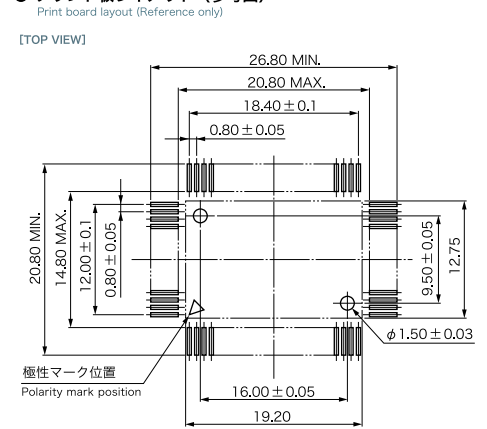
● プリント板レイアウト (参考図)
