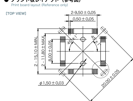
● プリント板レイアウト (参考図)
