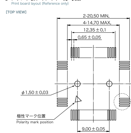
● プリント板レイアウト (参考図)
